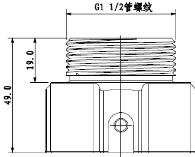
图3-3 快装接头尺寸（单位：mm）
