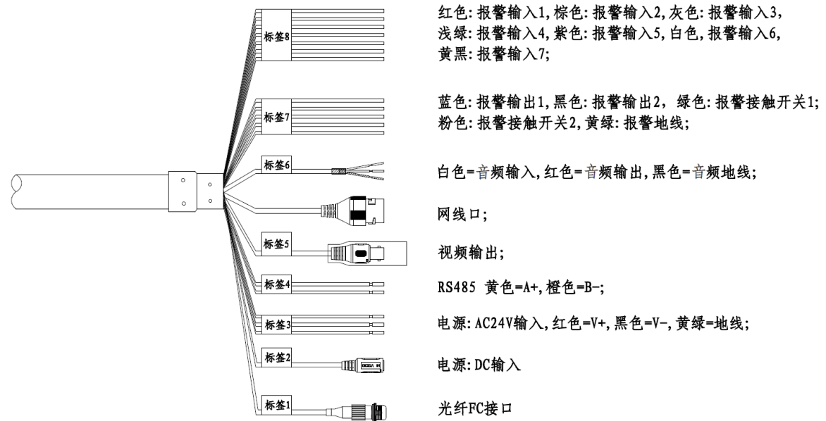
图2-4 线缆组成
