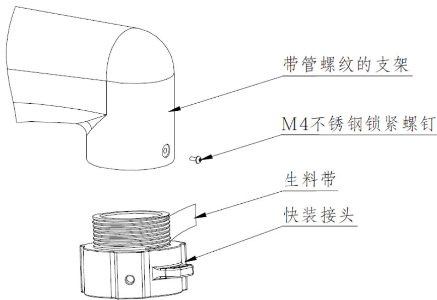
图2-3 安装快装接头示意图
